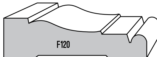
F120 - 3/4" X 2 1/2"
