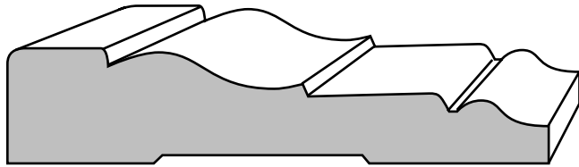
CASING F132 - 11/16" X 3 1/4"
