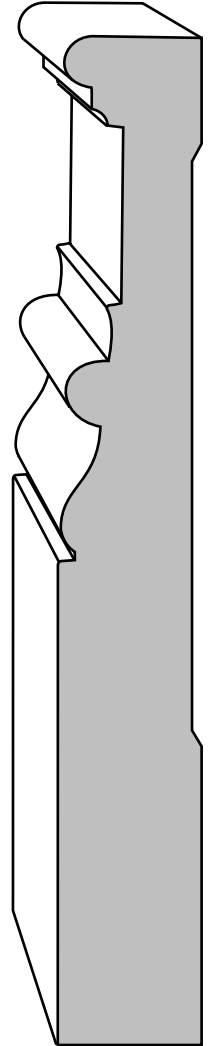
BASE F2450 - 11/16" X 5 1/4"
