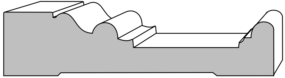
CASING F1450 - 1 1/16" X 4 1/2"
