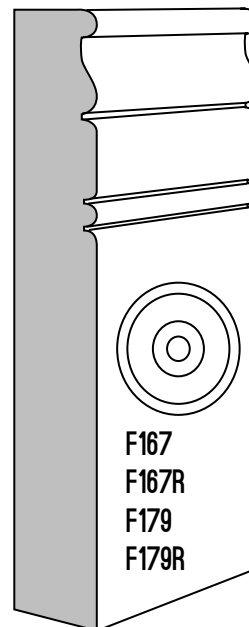
F167 - 1 1/16" X 3 1/2" X 8" F167R - 1 1/16" X 3 1/2" X 8"(W/ROSETTE) F179 - 1 1/16" X 6" X 8" F179R - 1 1/16" X 6" X 8"(W/ROSETTE)
