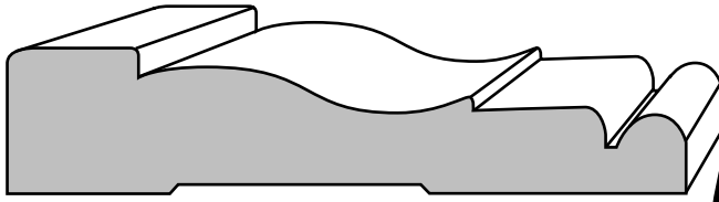
CASING F131 - 11/16" X 3 1/4"
