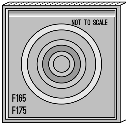
F165 - 1 1/16" X 3 1/2" X 3 1/2"(W/ROSETTE) F175 - 1" X 2 1/2" X 2 1/2"(W/ROSETTE)
