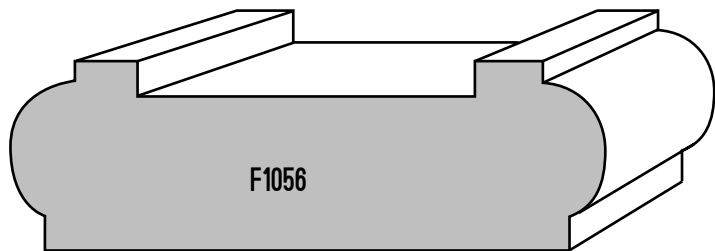
F1056 - 1" X 3 1/8" F1056FJ - 1" X 3 1/8"(FINGERJOINTED)
